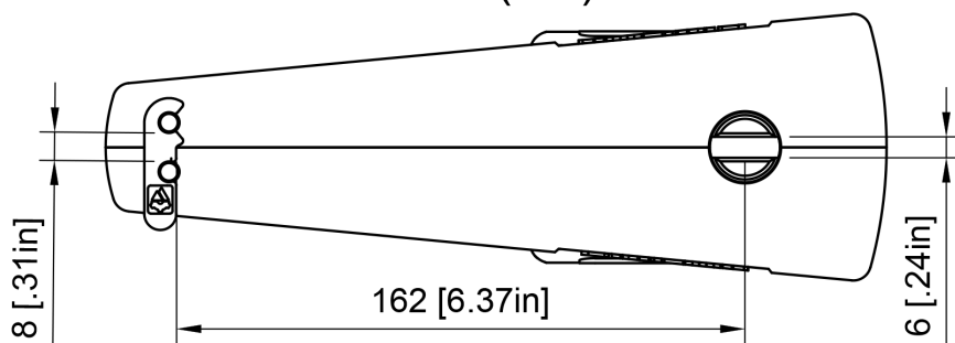
A-A (1:2)
